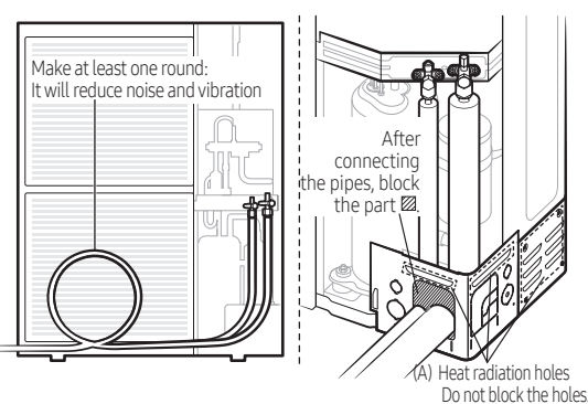
AC024/030/036/042/048XADCH
